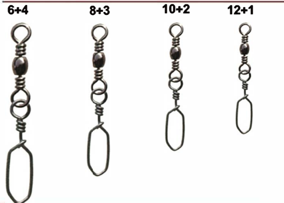
樽形轉環+方型別針 SL-1012 1:1
